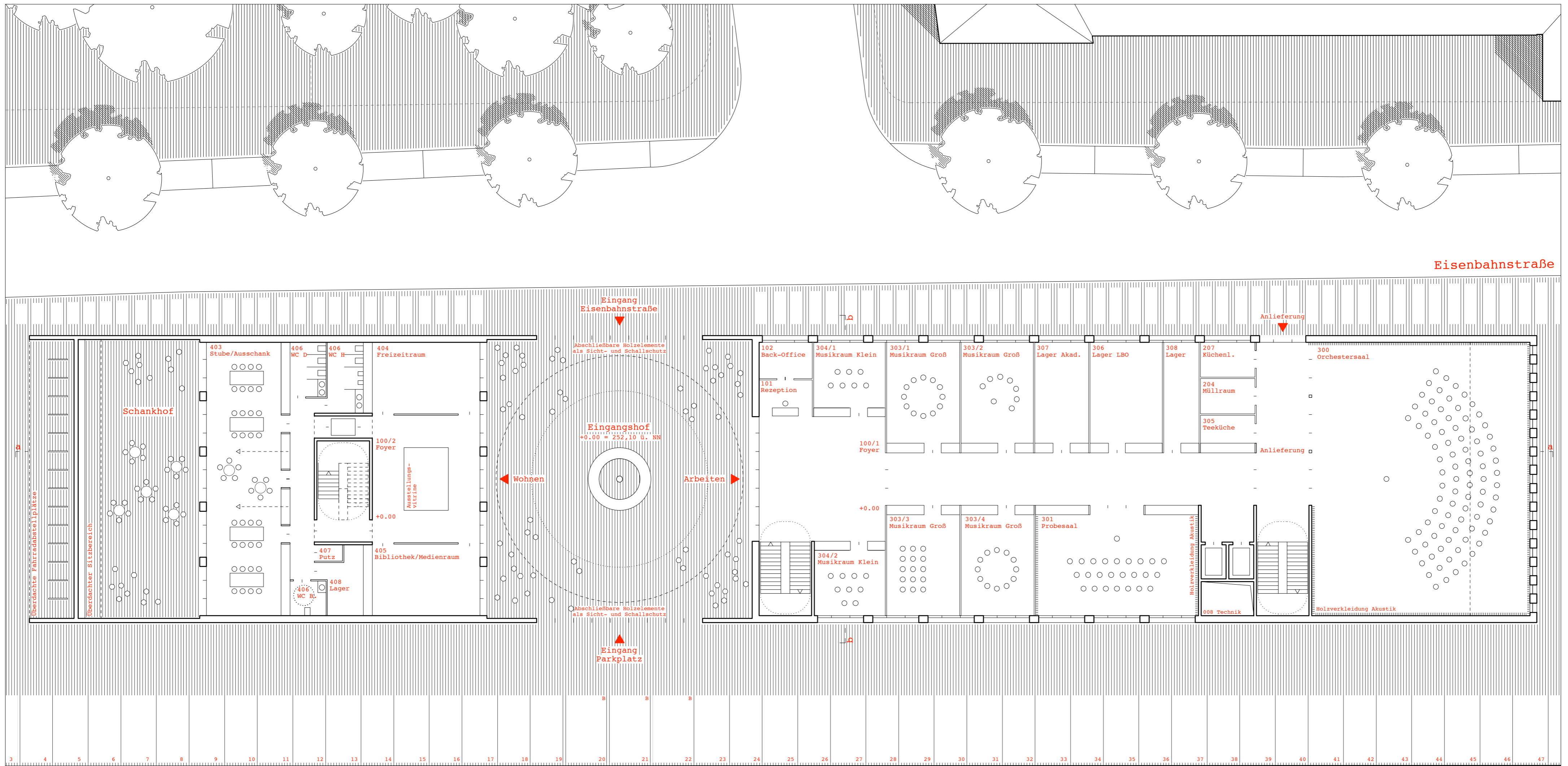
Grundriss Erdgeschoss
